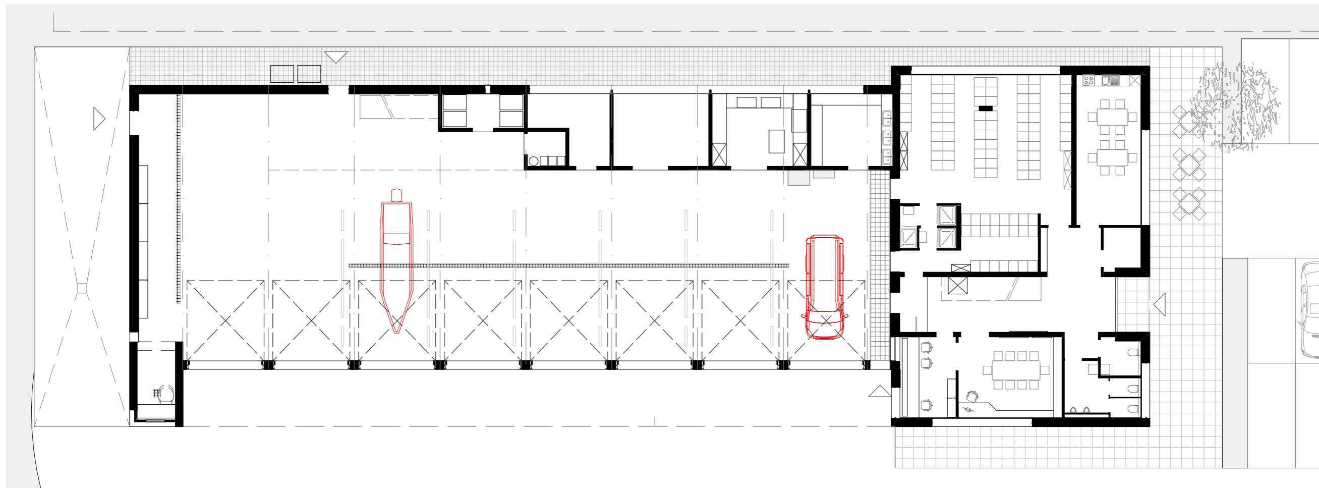
GRUNDRISS EG
