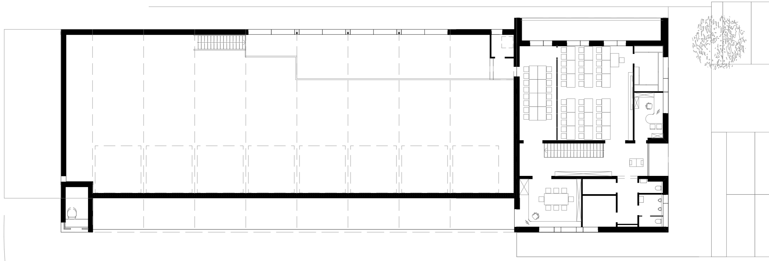
GRUNDRISS OG
